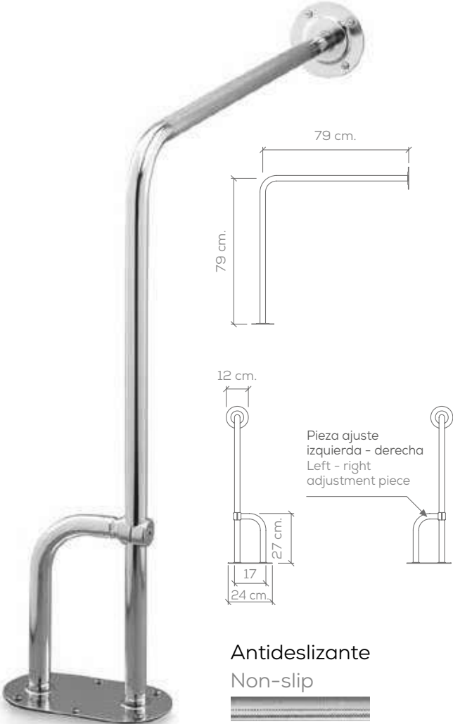
ASIDERO con apoyo auxiliar fijación suelo y pared inodoro. Pata ajustable a izquierda y derecha inox 18/10 Toilet handel with auxiliary support to install in floor and wall. Leg can be adjusted on the left and on the right 18/10 stainless steel
