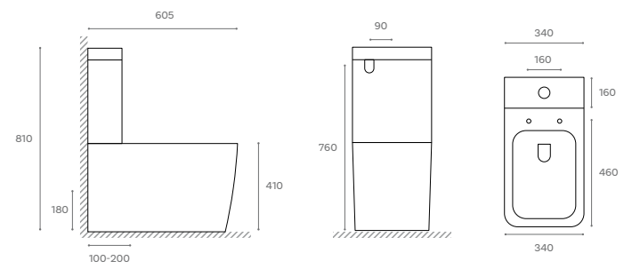
Inodoro. Toilette
