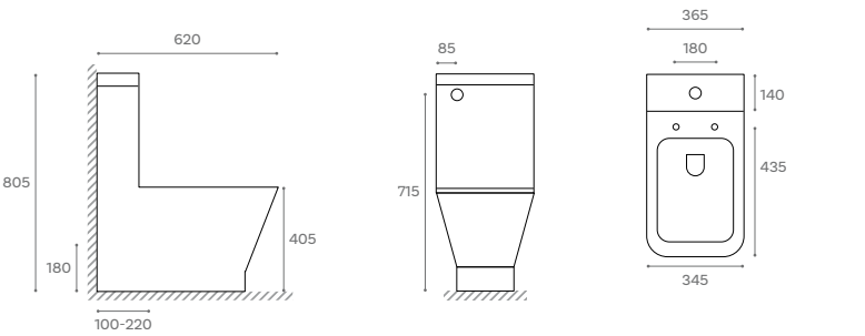
Inodoro. Toilette
