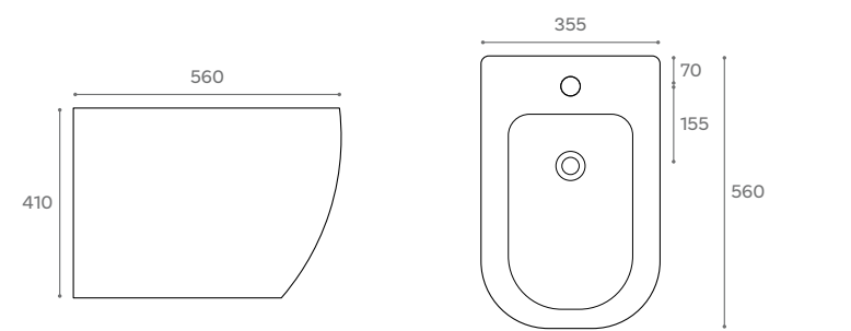
Bidé. Bidet
