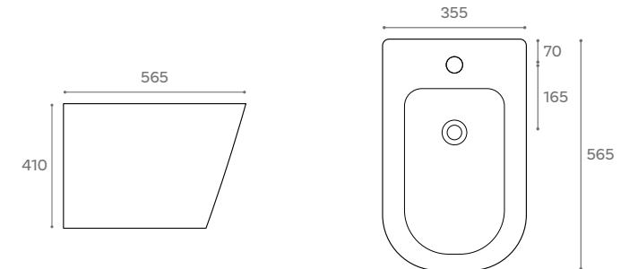
Bidé. Bidet
