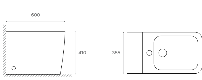
Bidé. Bidet
