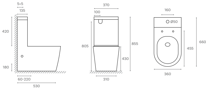
Inodoro. Toilette
