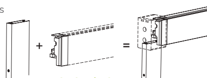
Dibujo técnico Complemento GS604
