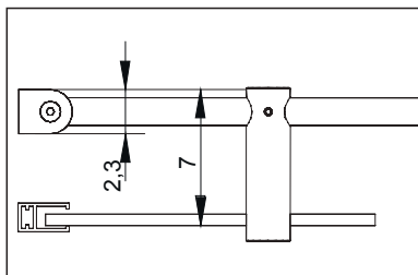
Detalle fijación barra a pared
