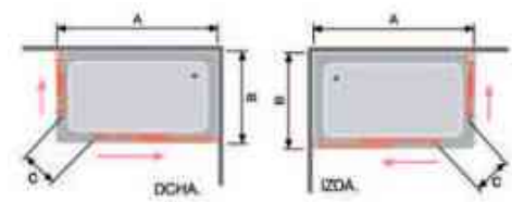
Dibujo técnico GS607 + GS607 Angular de Ducha
