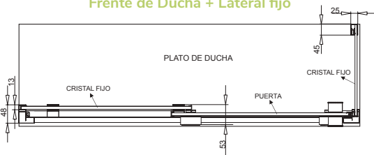
Dibujo técnico VO102 + VO103 Frente de Ducha + Lateral fijo
