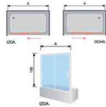
Dibujo técnico SU152 Frente de ducha
