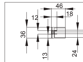
Dibujo técnico SU107 Frente de ducha
