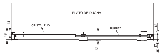
Dibujo técnico VO102 Frente de Ducha con perfil de cierre
