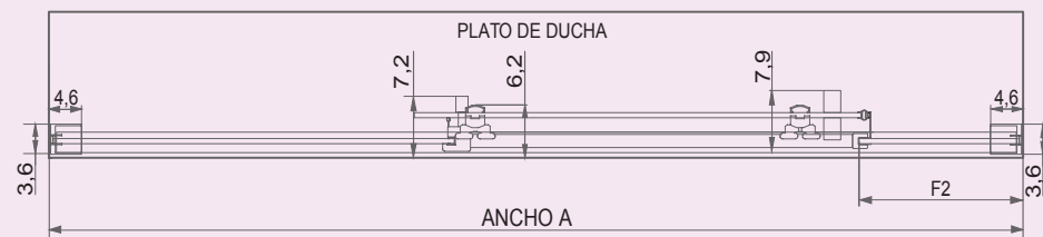
Dibujo técnico SU107
